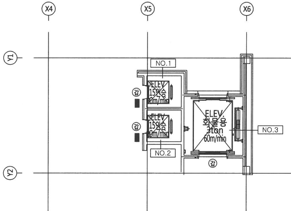
승강기 배치도
