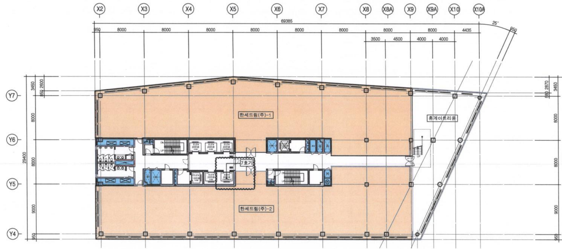
2 11층 평면도 축척: 1/400
