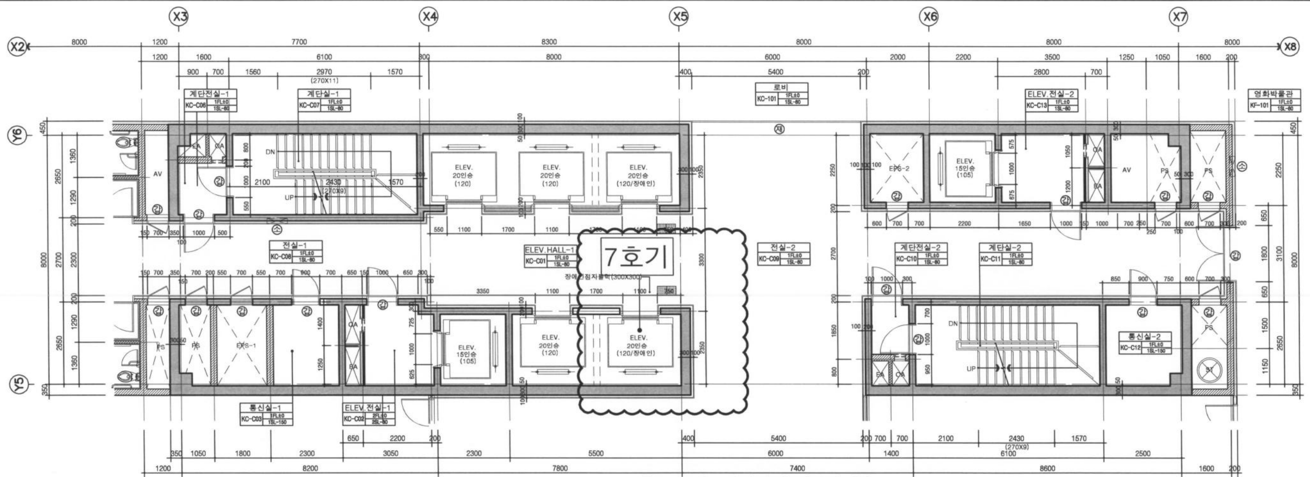
1 코아-1평면상세도(지상1층) 축척:1/60
