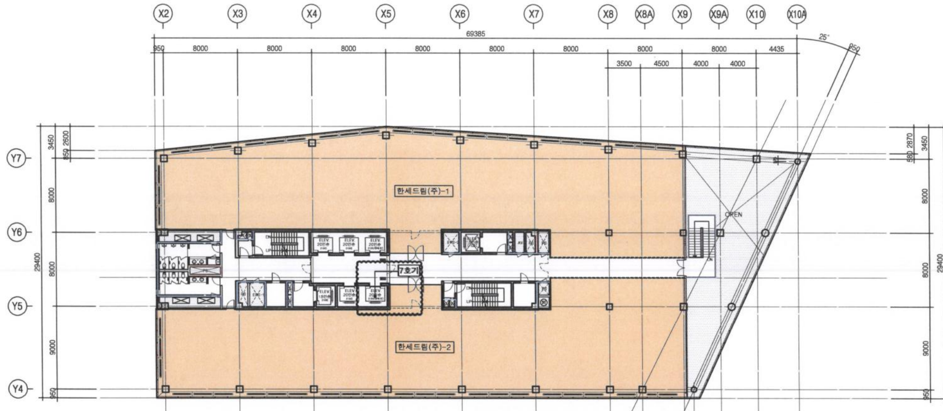
2 12층 평면도 축척: 1/400
