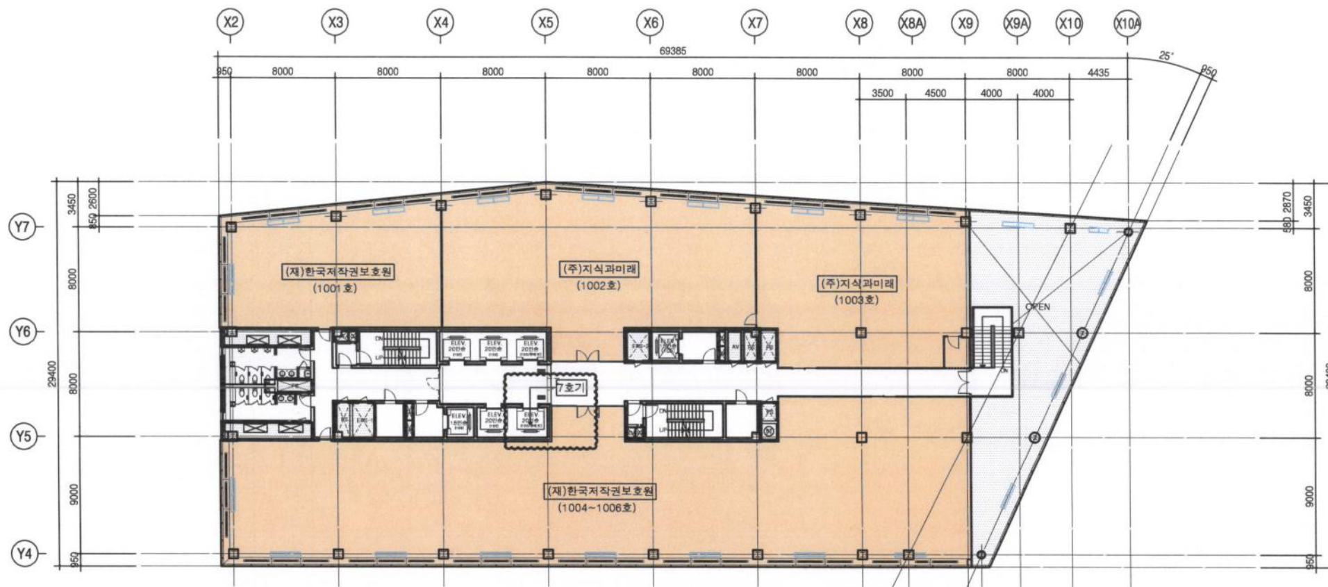
1 10층 평면도 축척: 1/400
