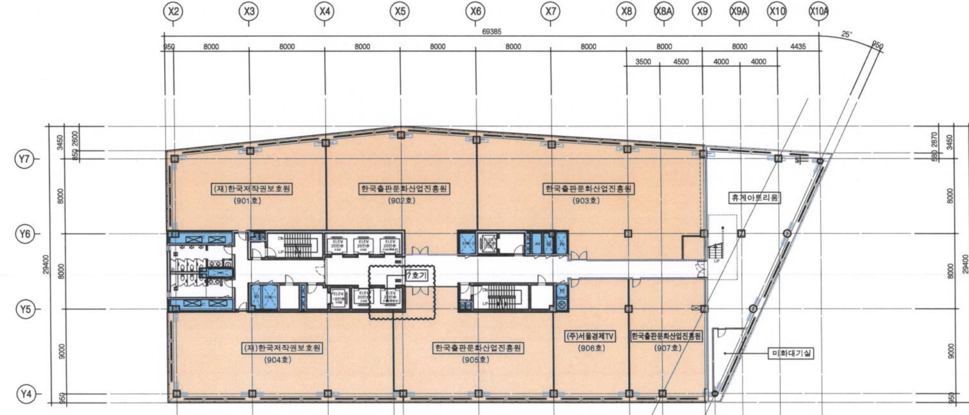
2 9층 평면도 축척: 1/400
