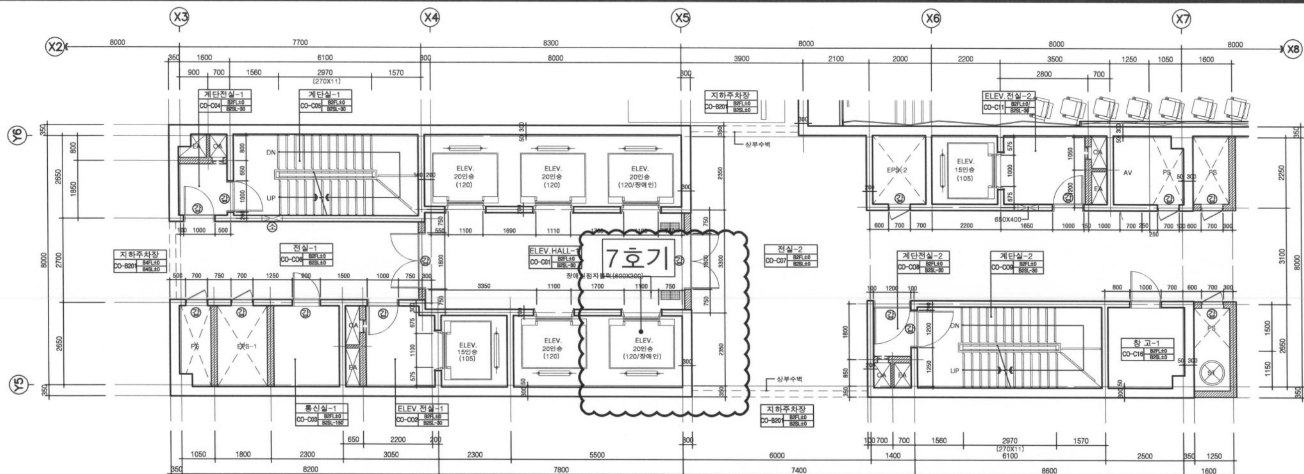
1 코아-1평면상세도(지하2층) 축척:1/60
