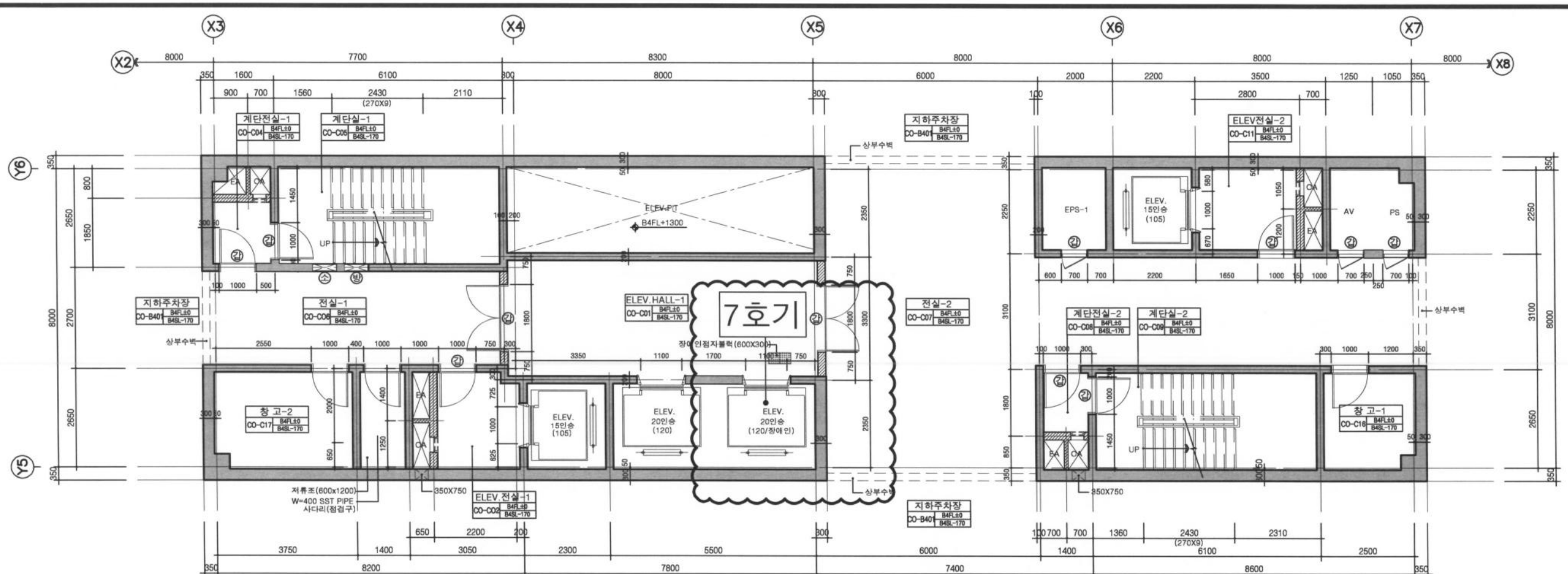
1 코아-1평면상세도(지하4층) 축척:1/60
