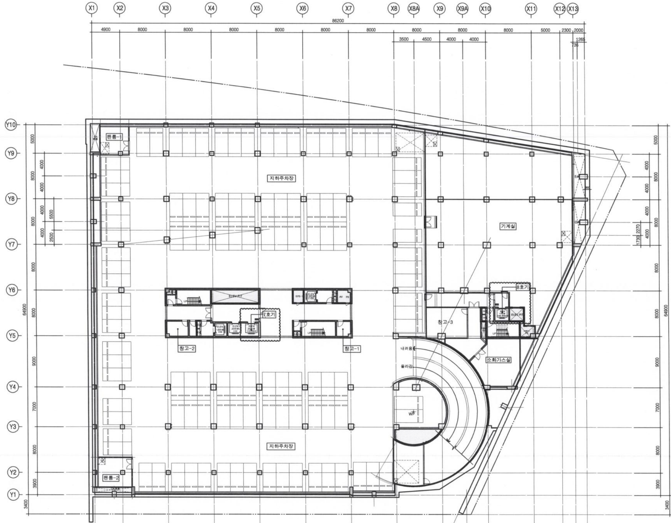
1 지하 4층 평면도 축척: 1/400
