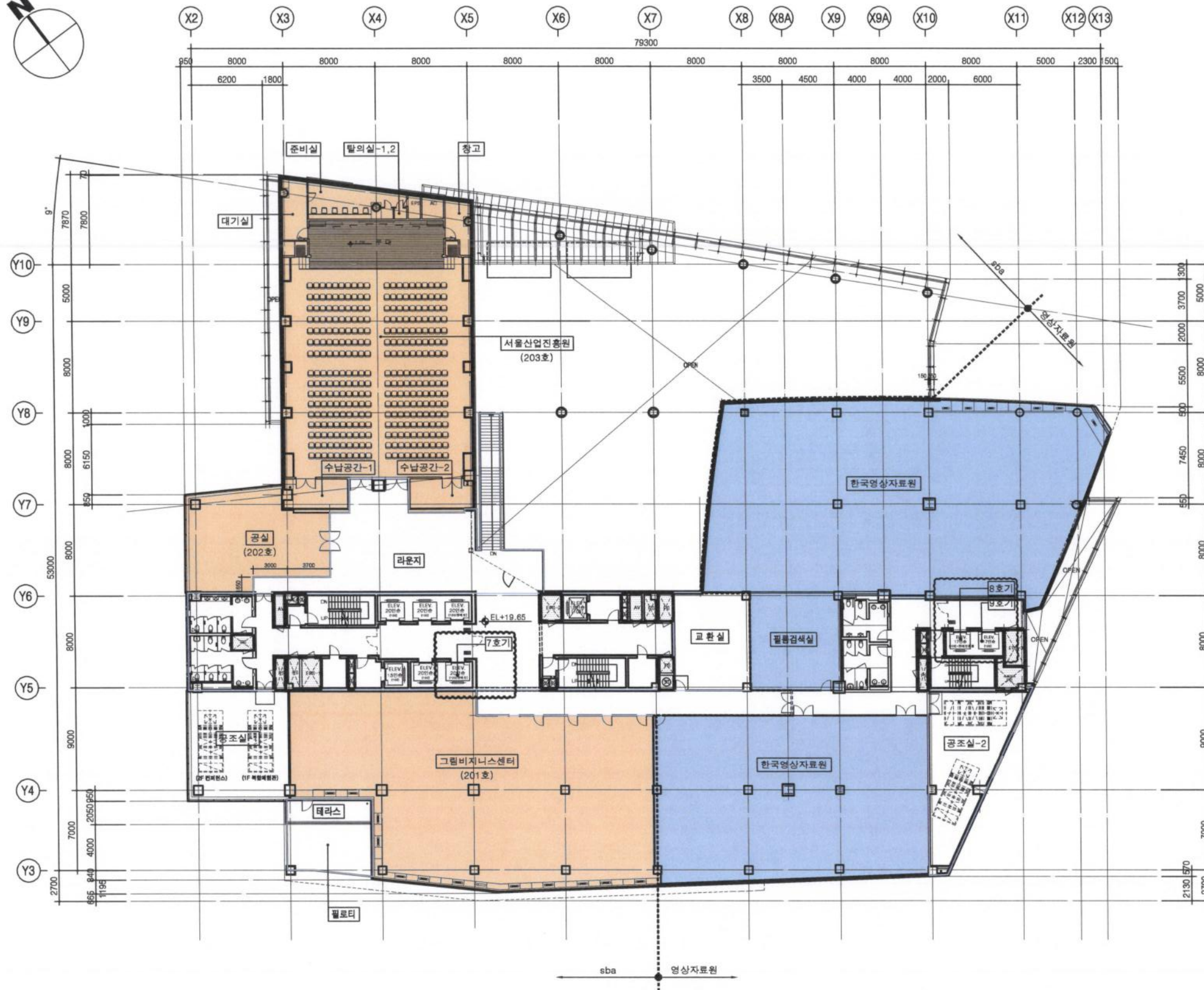
1 2층 평면도 축척: 1/400
