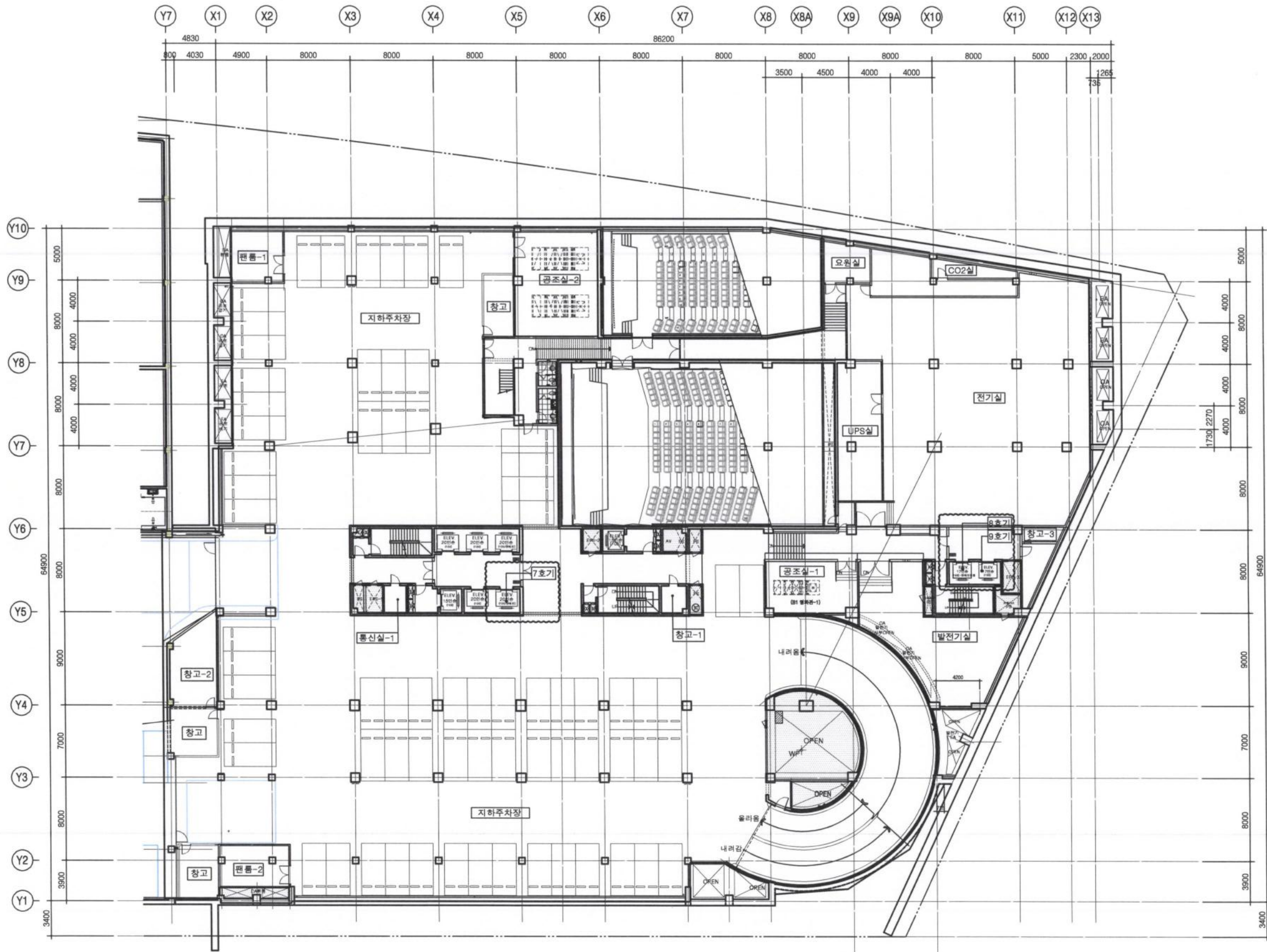
1 지하 2층 평면도 축척: 1/400
