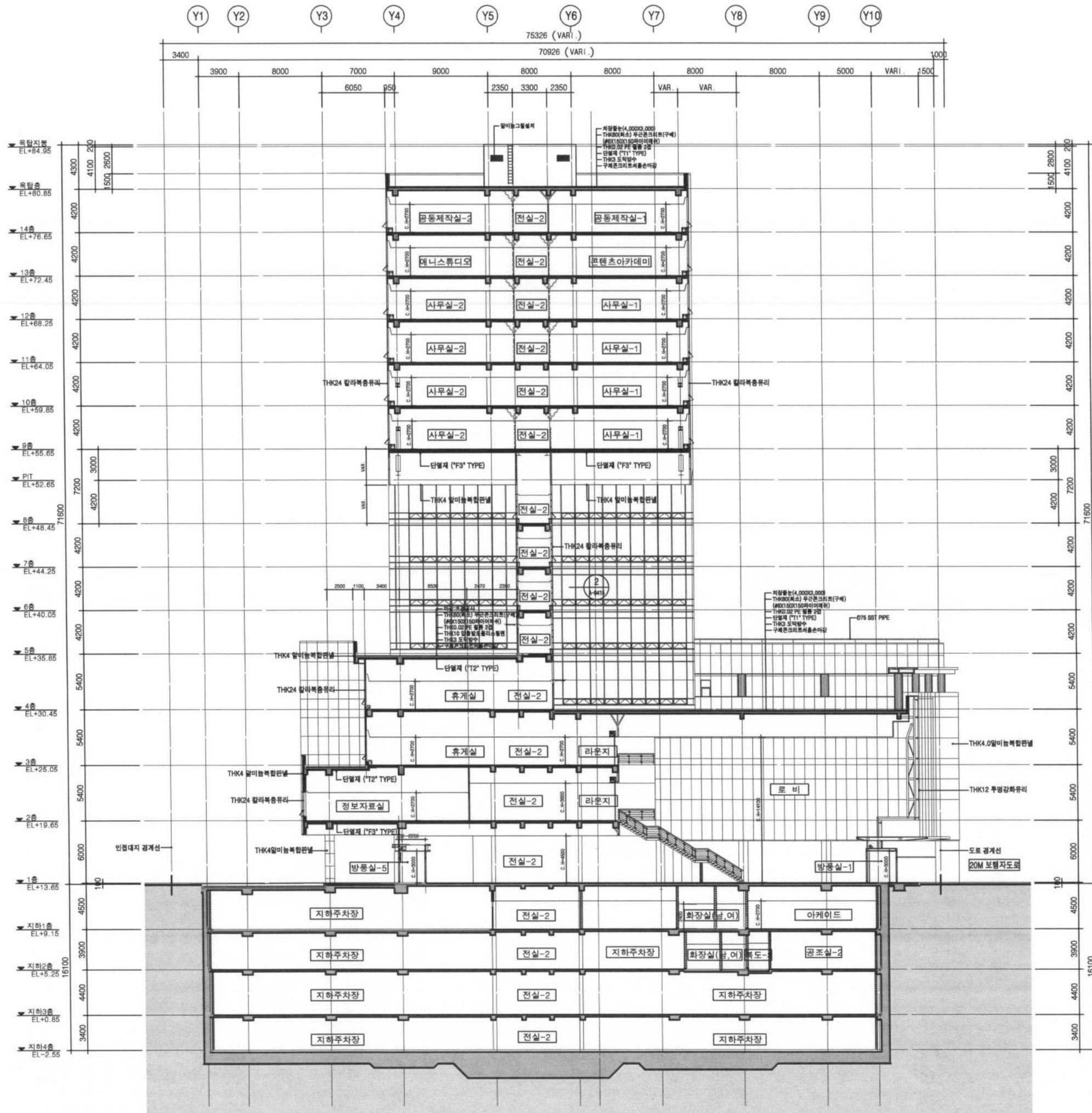
1 주 단 면 도-2 축척: 1/200
