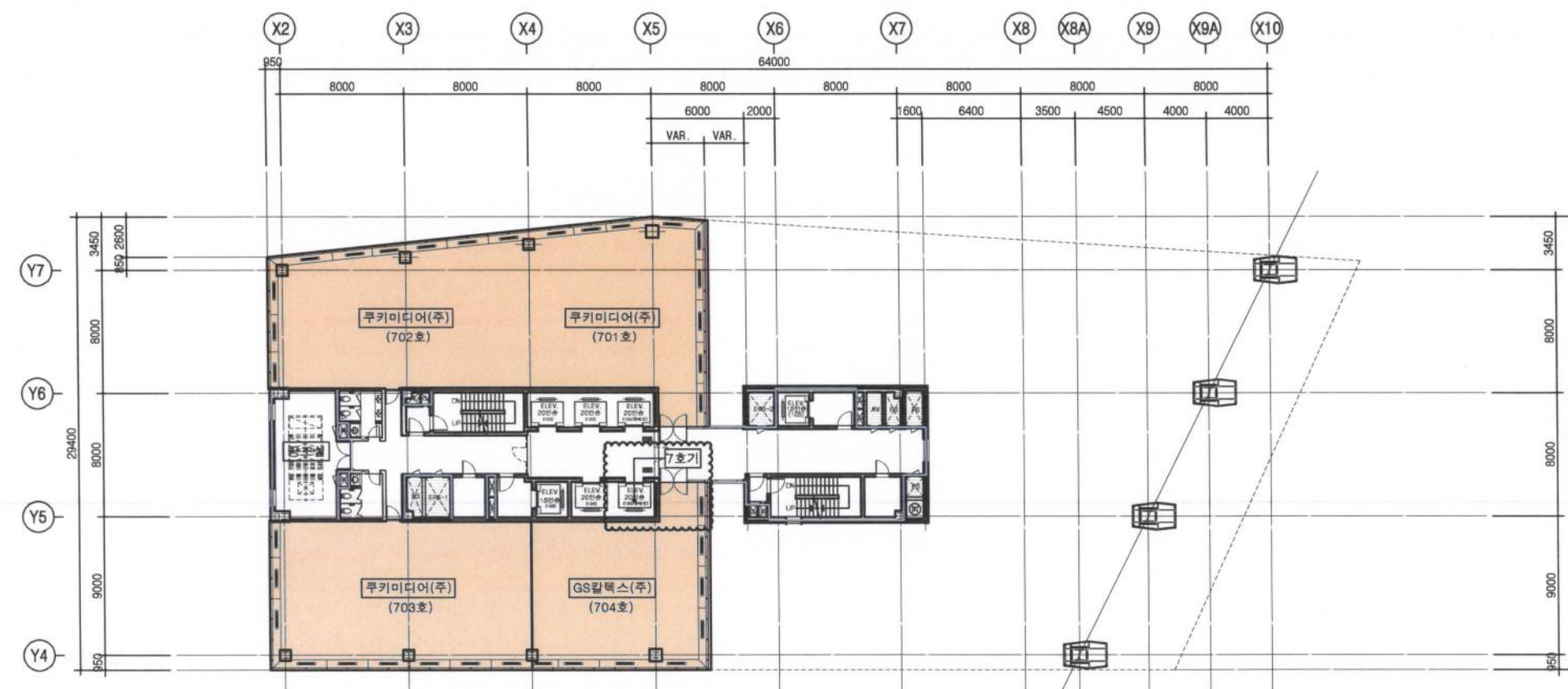
2 7층 평면도 축척: 1/400
