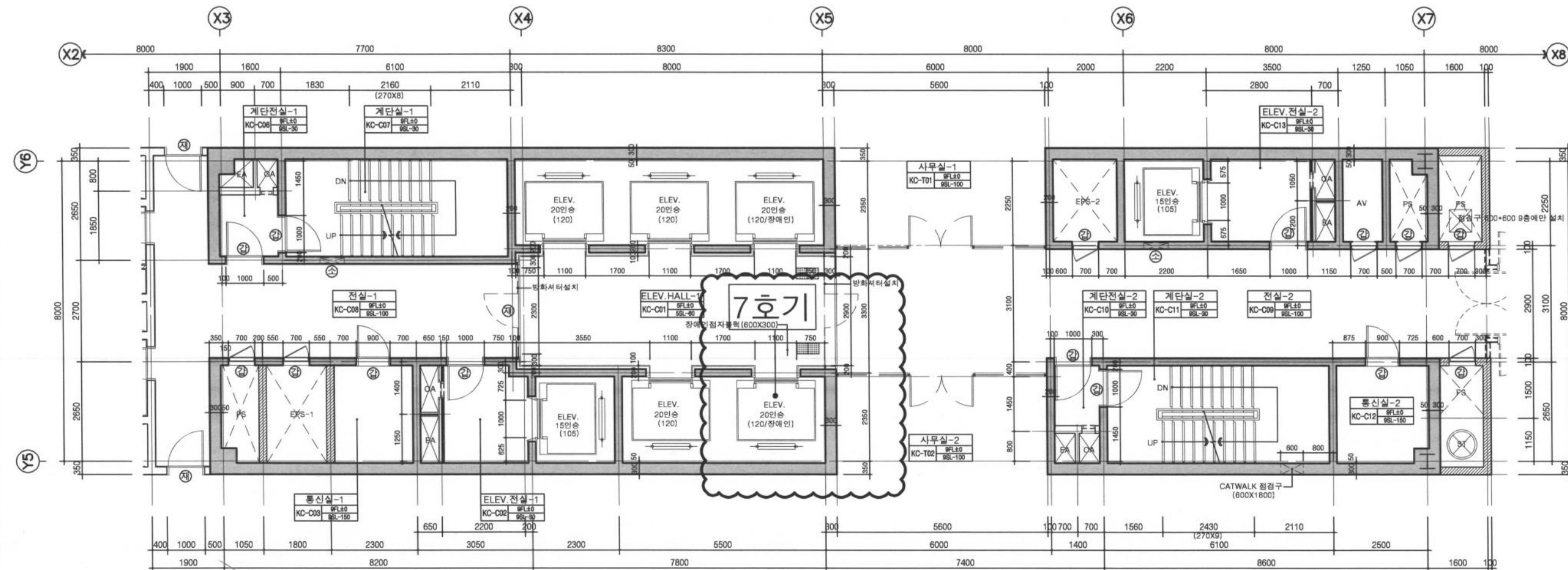
2 코아-1 평면상세도(지상9~13층) 축척: 1/60
