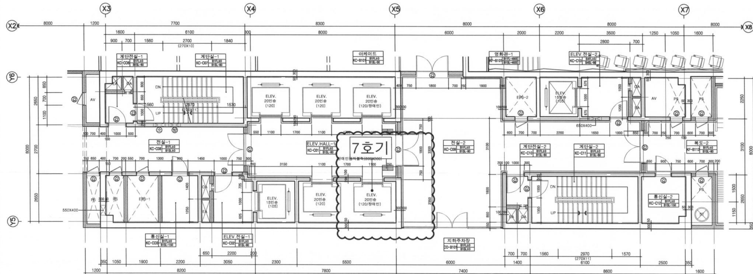
2 코아-1평면상세도(지하1층) 축척:1/60
