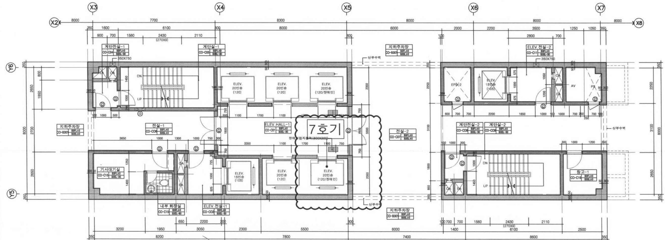
2 코아-1평면상세도(지하3층) 축척:1/60
