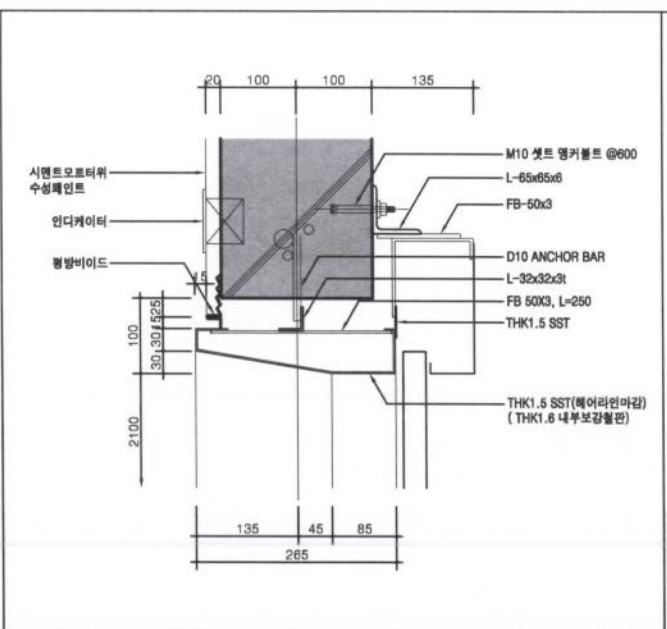
H 2 HEAD(지하4~지하2층 / ELEV. 전실-1,2) 축척 : 1/5
