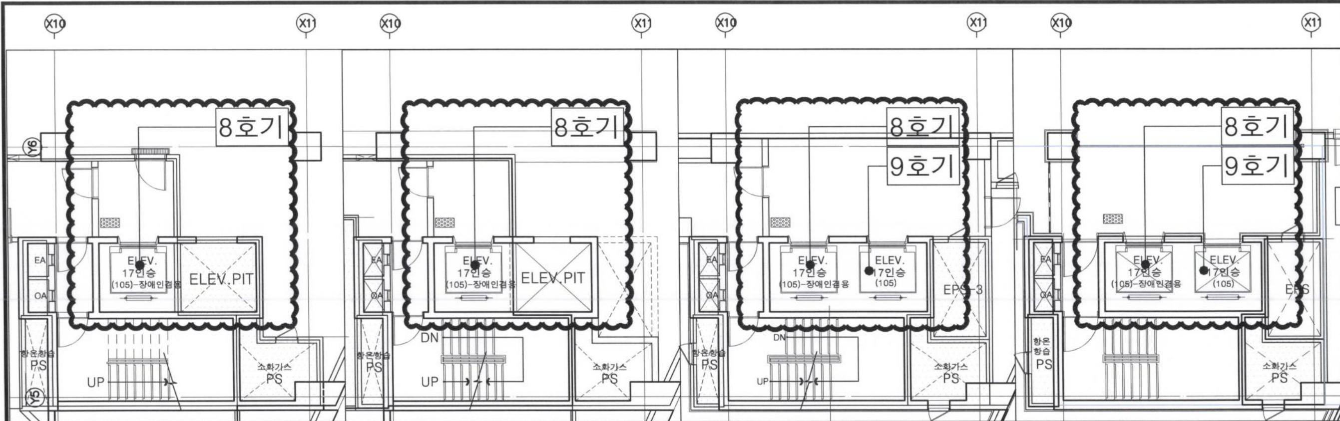
1 코아-2평면상세도(지하4층) 축척:1/60
