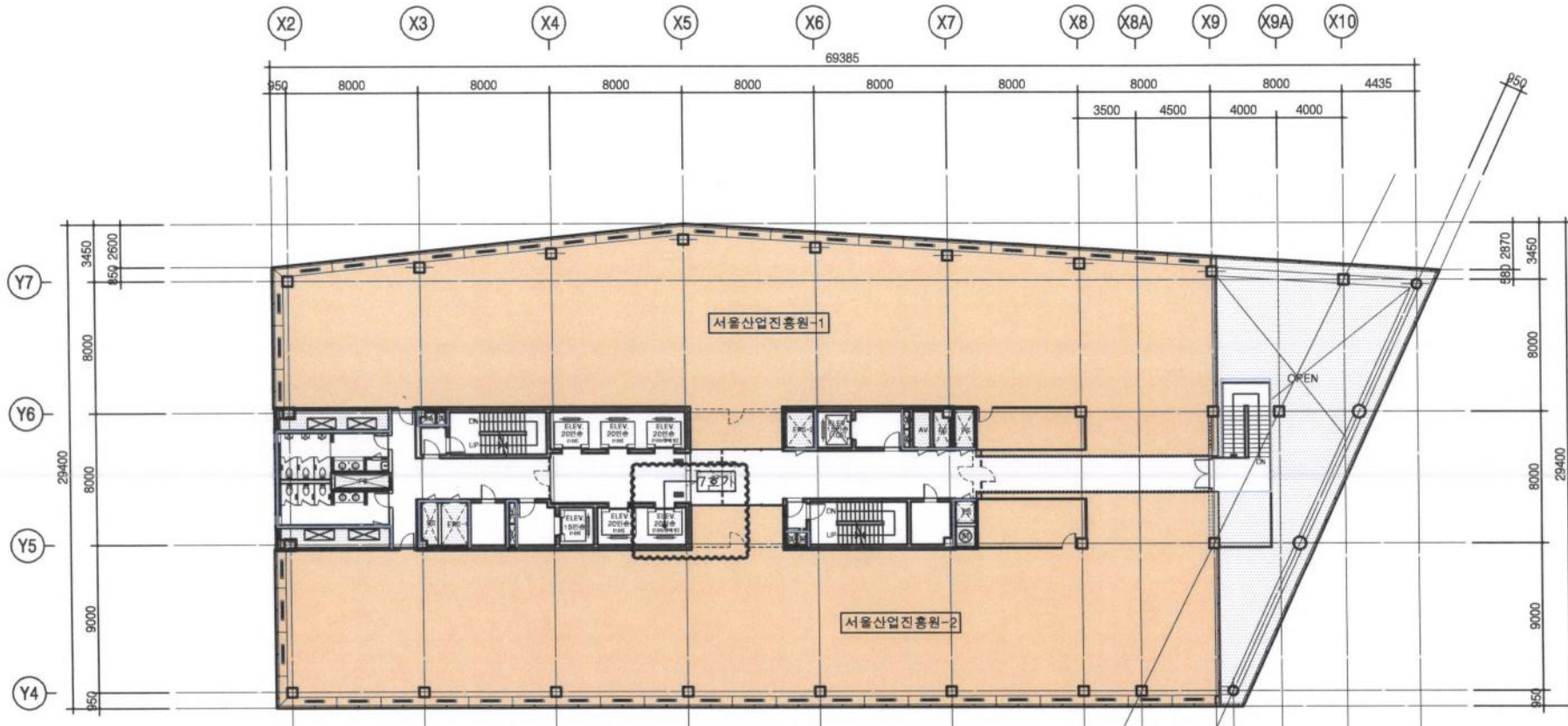
1 14층 평면도 축척: 1/400
