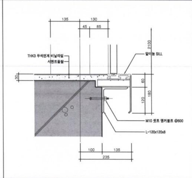
S 2 SILL(지하4~지하2층 / ELEV. 전실-1,2) 축척 : 1/5
