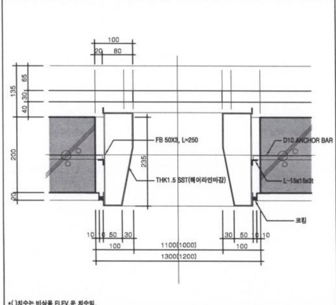
J 2 JAMB(지하4~지하2층 / ELEV. 전실-1,2) 축척 : 1/5
