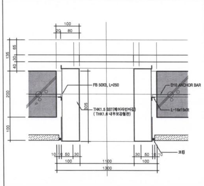
J 1 JAMB(ELEV. HALL-1,2 지하1~14층) 축척 : 1/5
