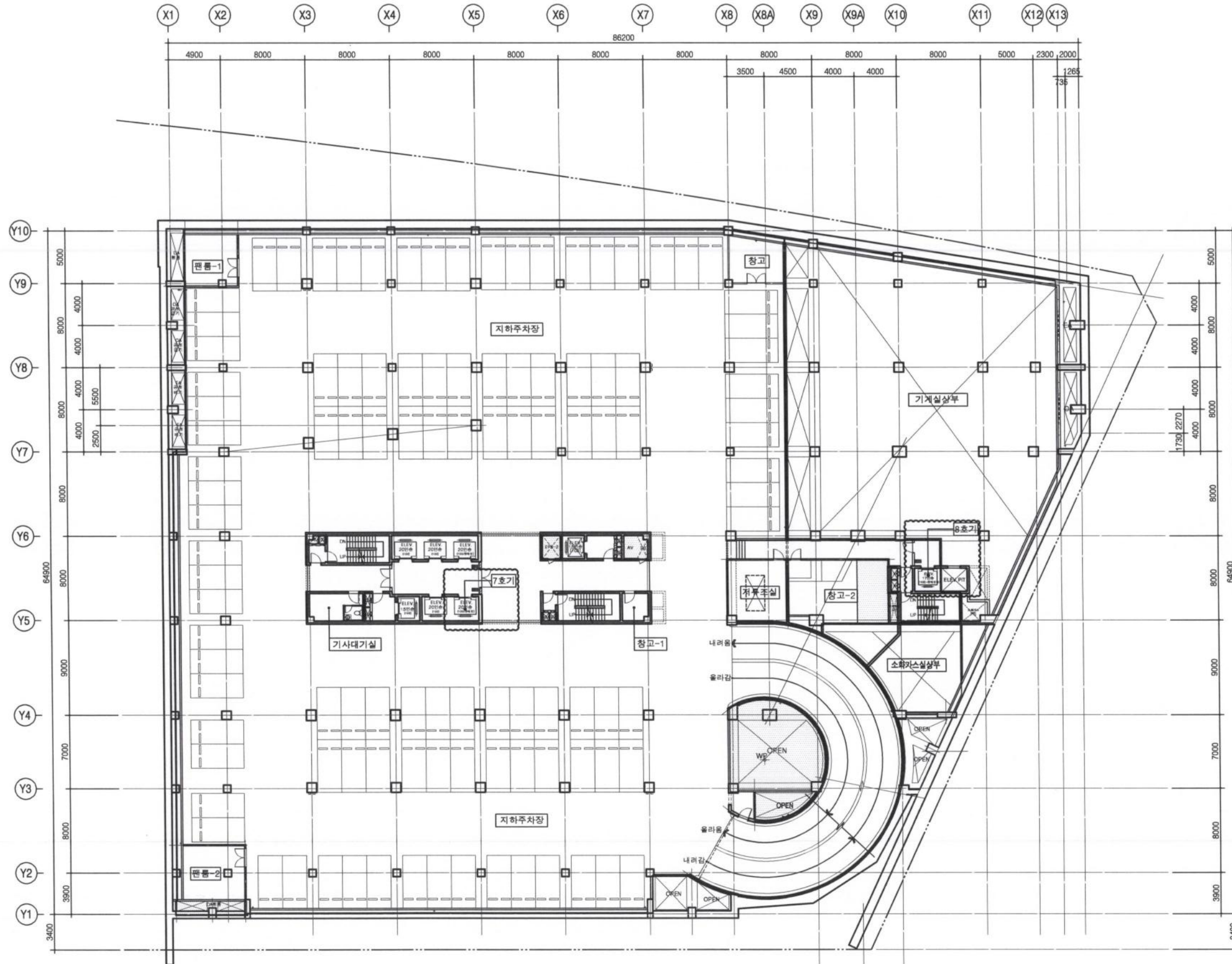
1 지하 3층 평면도 축척: 1/400
