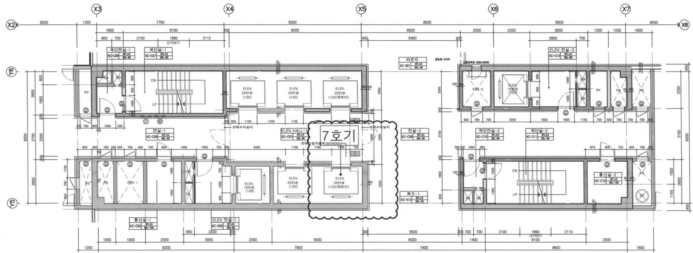
2 코아-1평면상세도(지상2~3층) 축척:1/60
