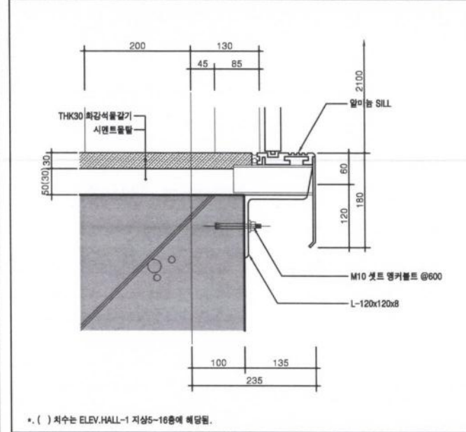
S 1 SILL(ELEV. HALL-1,2 지하1~14층) 축척 : 1/5
