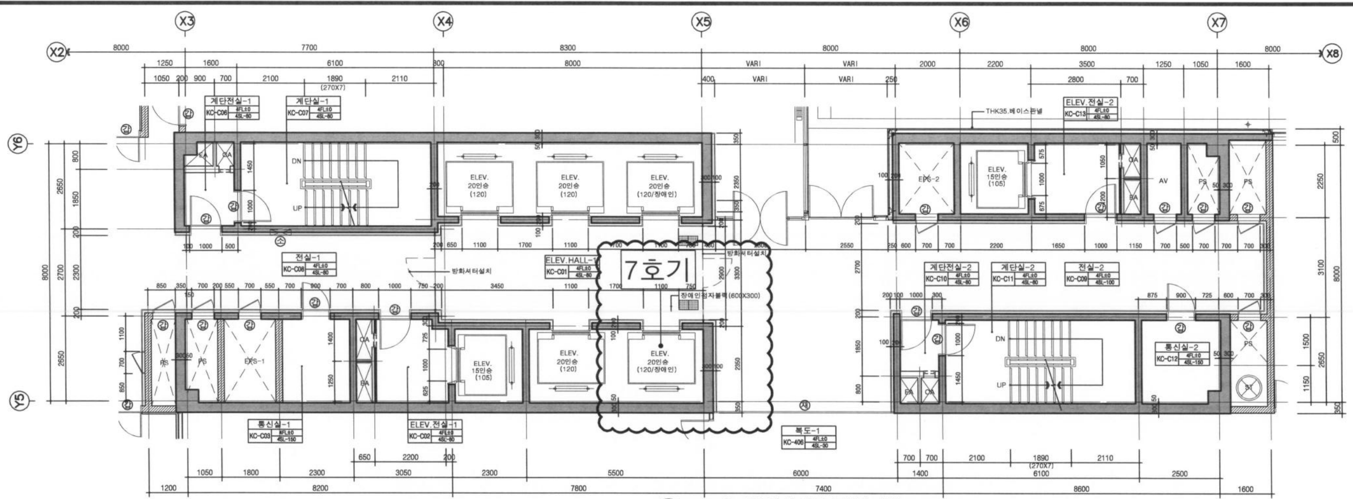
1 코아-1평면상세도(지상4층) 축척: 1/60
