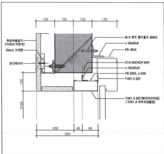
H 1 HEAD(ELEV. HALL-1,2 지하1~14층) 축척 : 1/5
