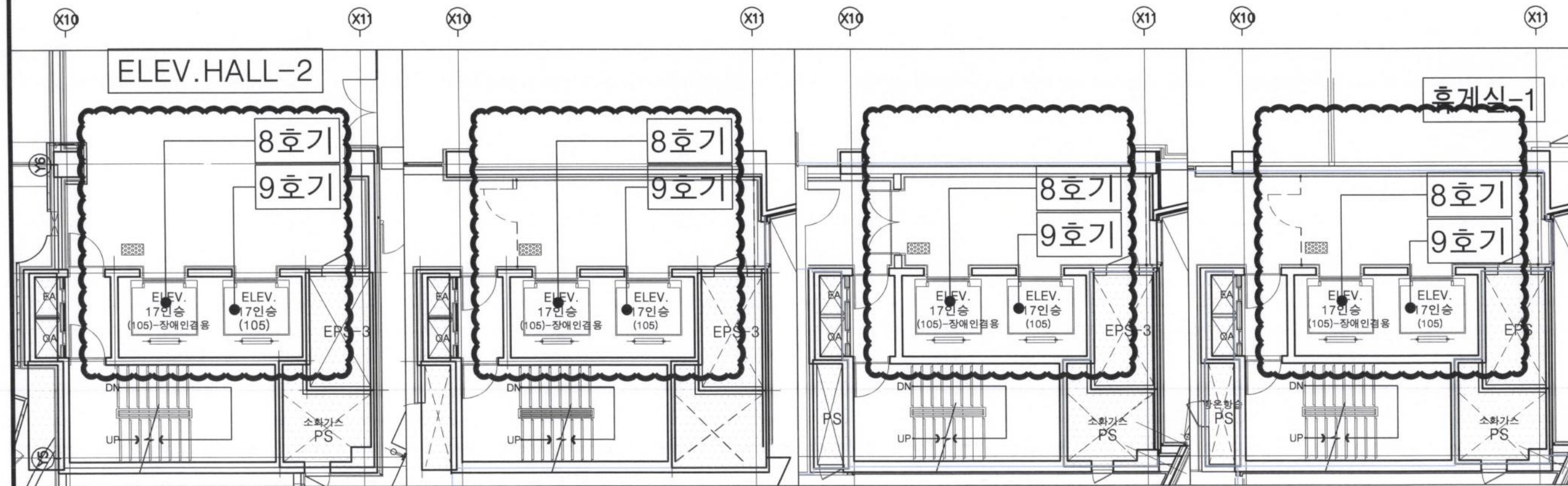
1 코아-2평면상세도(지상1층) 축척:1/60
