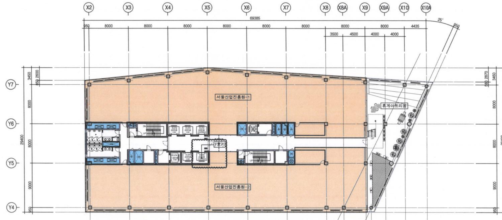
1 13층 평면도 축척: 1/400
