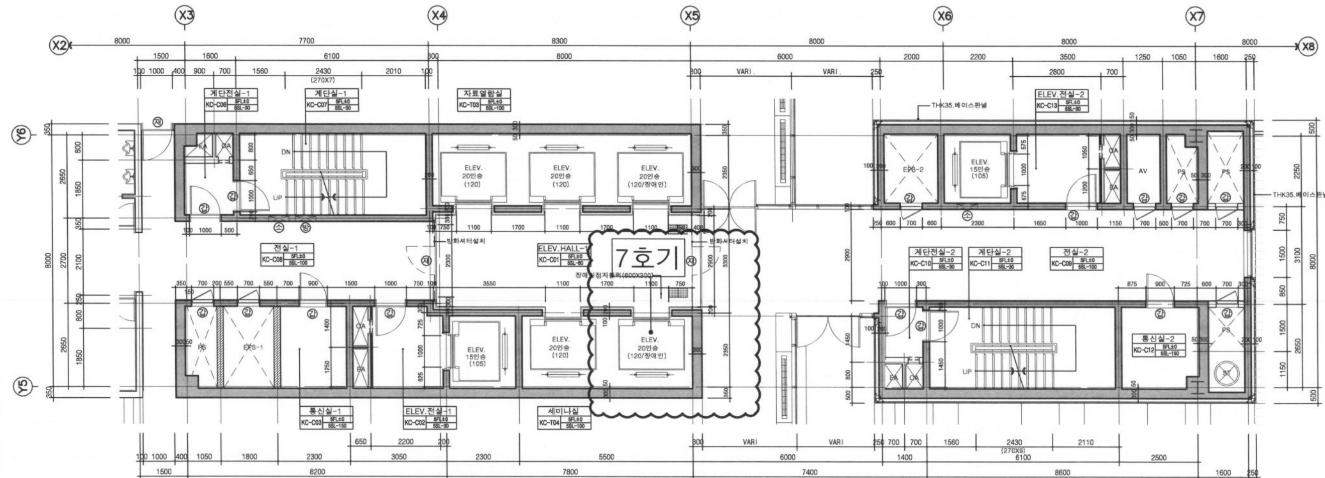
1 코아-1평면상세도(지상5층) 축척: 1/60
