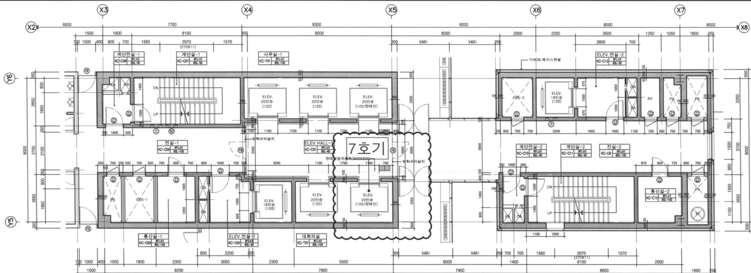
1 코아-1 평면상세도(지상6~8층) 축척: 1/60
