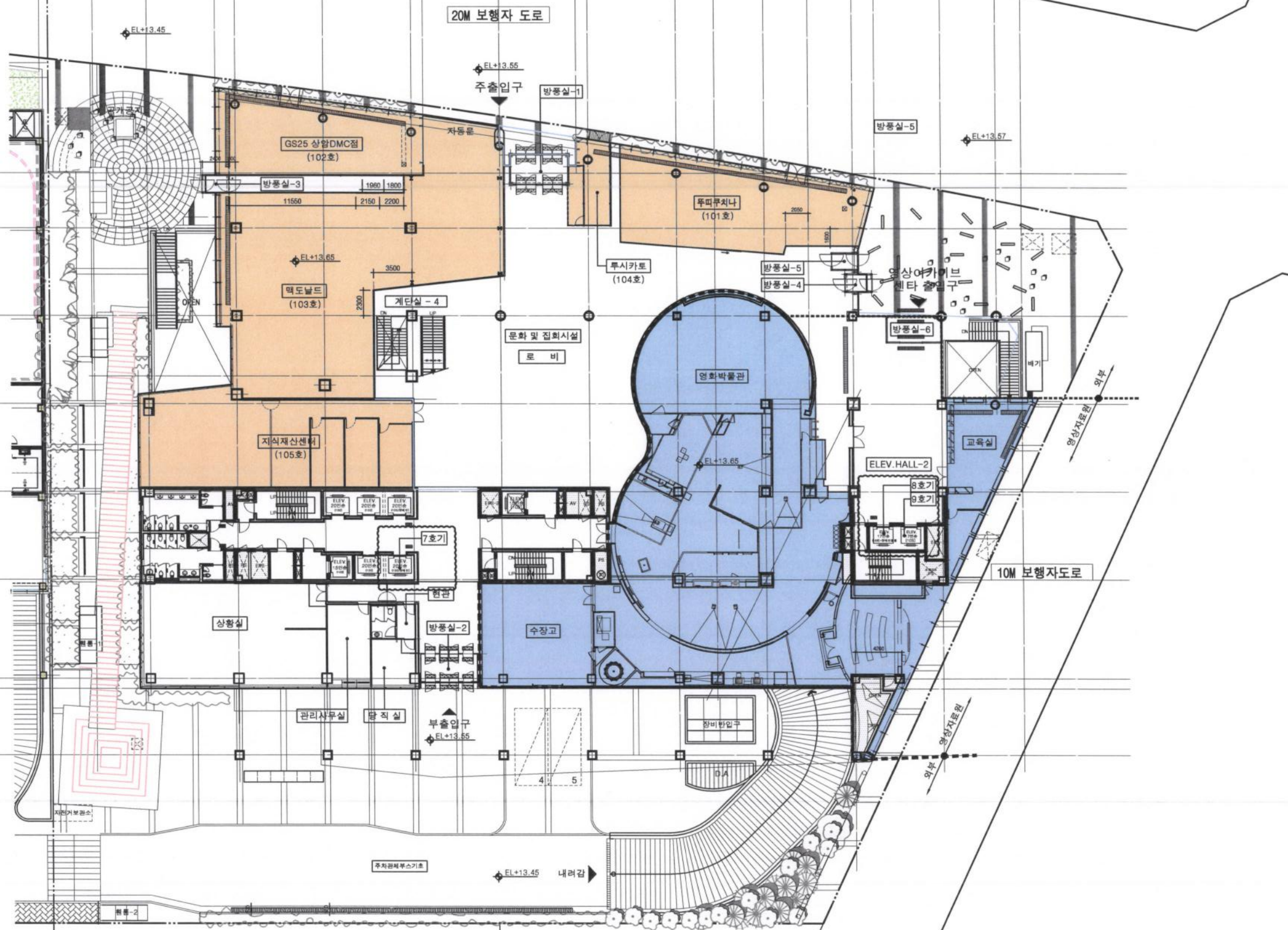
1 1층 평면도 축척: 1/400
