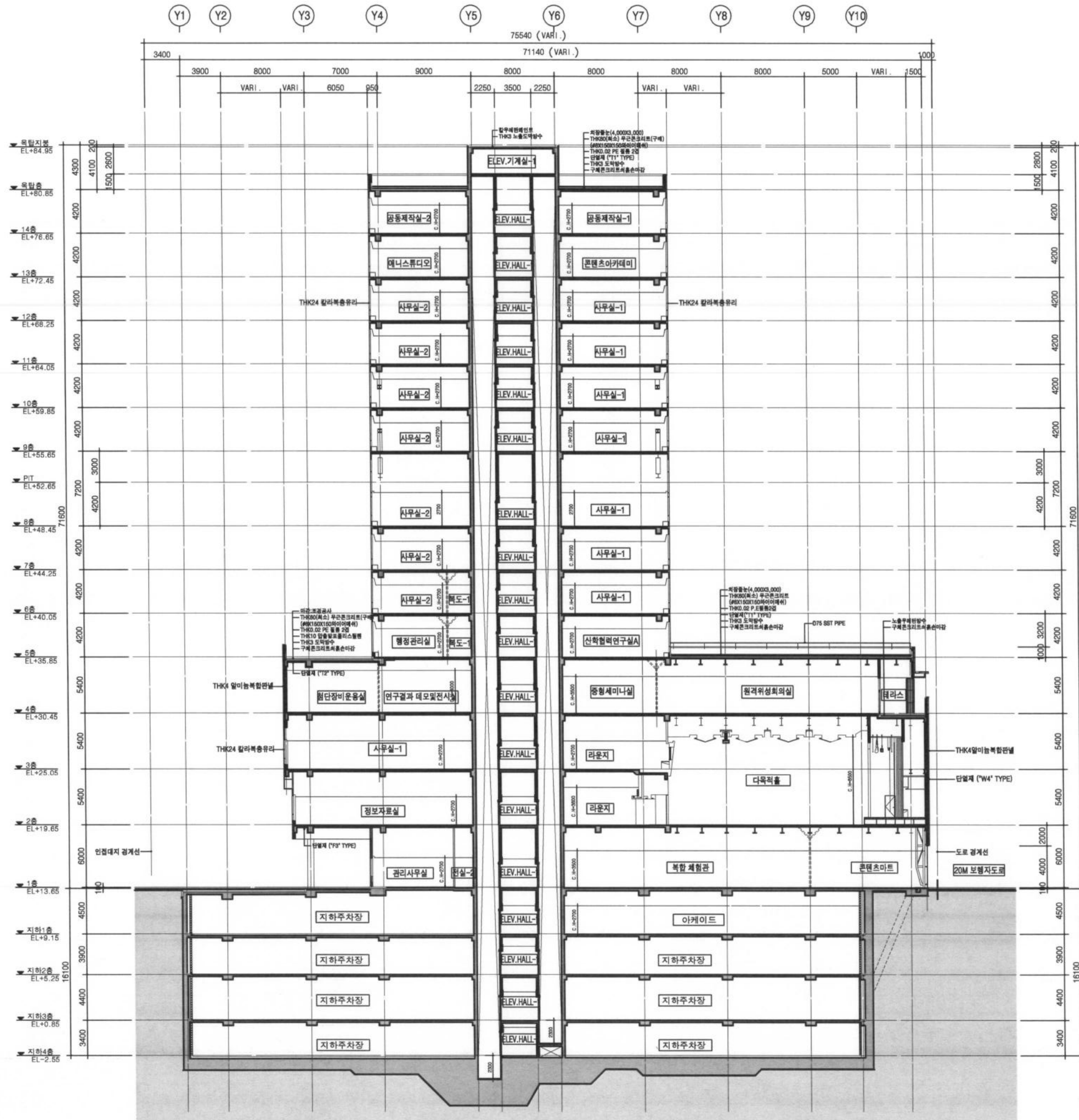
1 주 단 면 도-1 축척: 1/200
