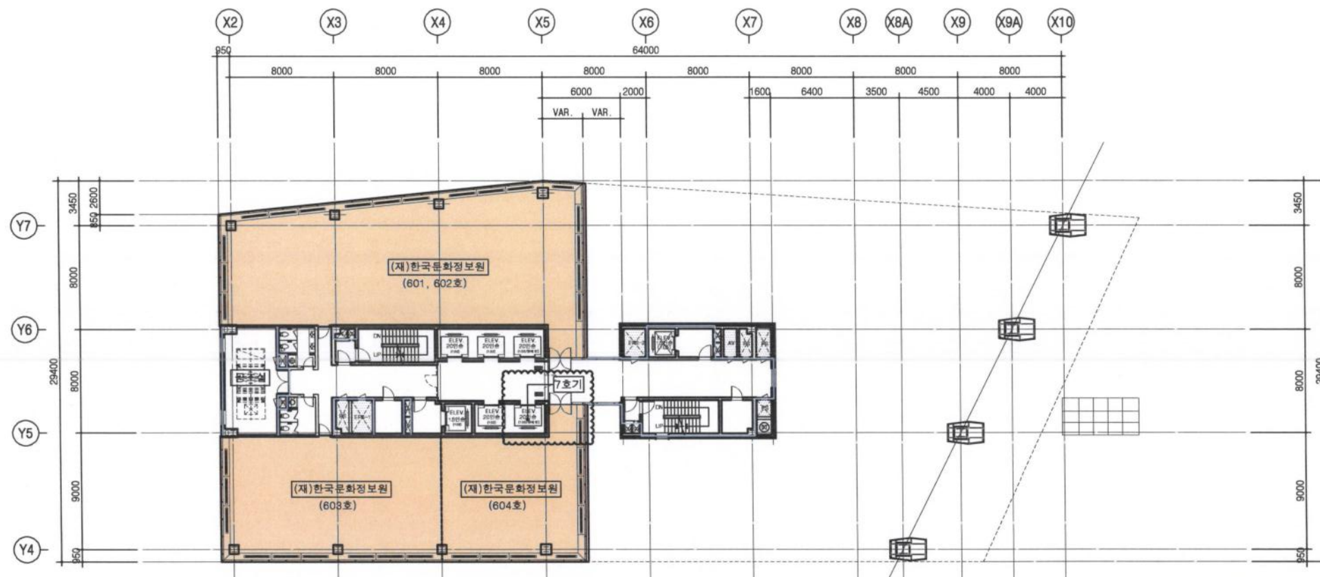
1 6층 평면도 축척: 1/400
